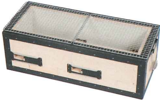
No.6128 22号 L-930×W350×H200mm No.6127 17号 L-700×W350×H200mm No.6126 12号 L-470×W350×H200mm No.6123 8F号 L-310×W230×H200mm No.6122 55号 L-270×W170×H130mm
